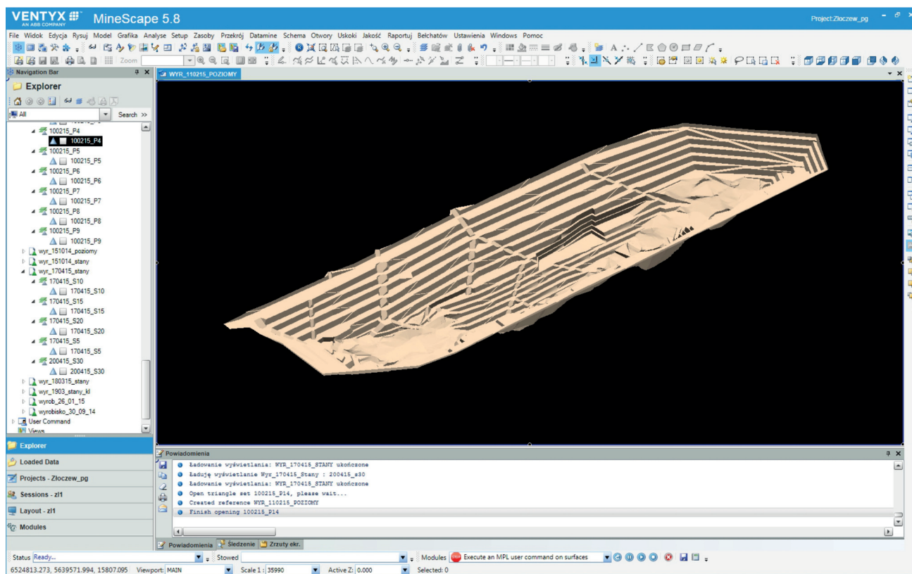
Rys. 4. Model wyrobiska projektowanego w systemie MineScape
