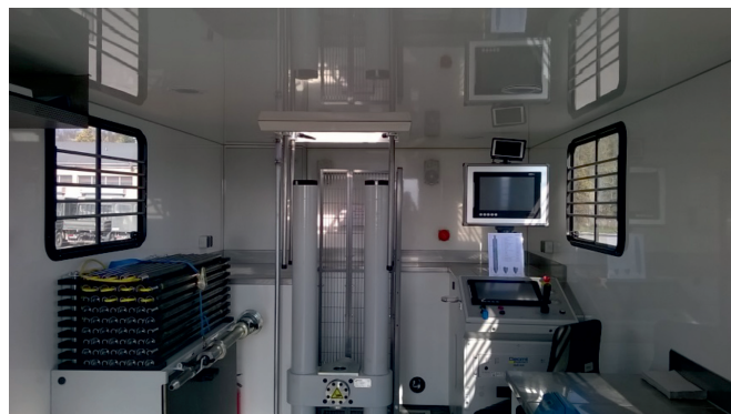
Fot. 2. Wnętrze sondy statycznej GRIZZLY 200 kN
