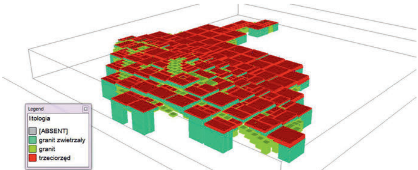
Rys. 5. Strukturalny model blokowy złoża granitu Fig. 5. Granite deposit structural block model
