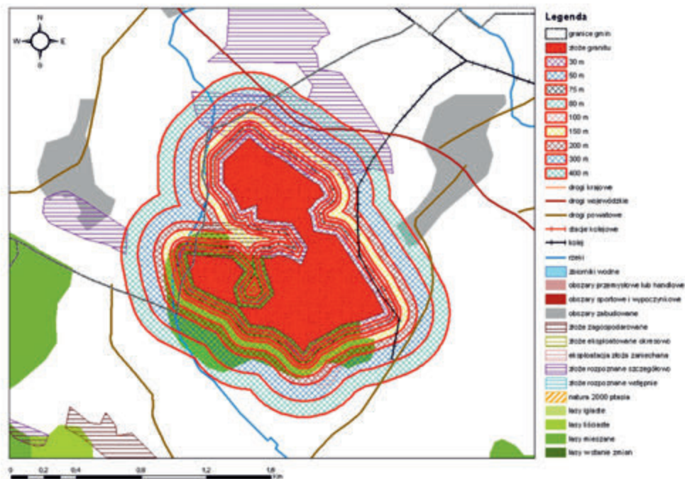
Rys. 4. Wielkość strefy zagrożenia dla obiektów ze względu na drgania sejsmiczne przy strzelaniu w otworach wiertniczych Fig. 4. Danger zone size for objects due to boreholes blasting seismic vibrations
