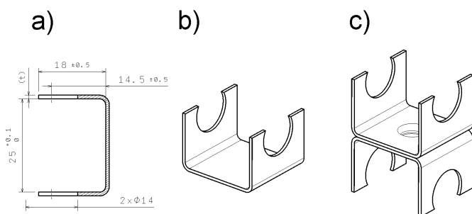
Rys. 5. Próbką do badań złącza: a) przekrój; b) widok izometryczny komponentu; c) widok izometryczny gotowej próbki
