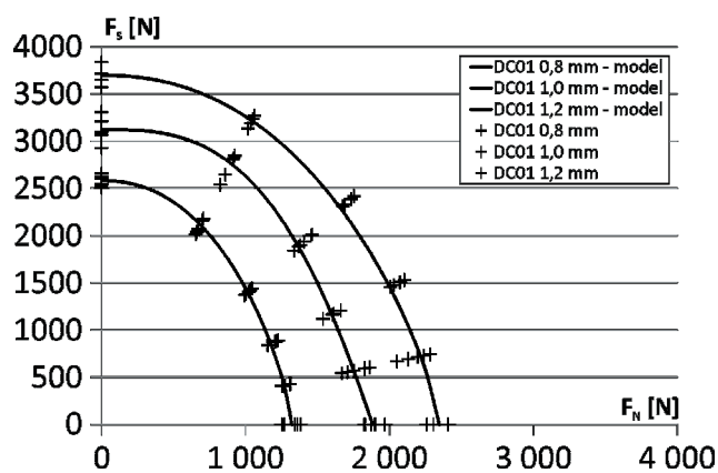
Rys. 6. Dopasowanie modelu do danych pomiarowych – DC01
