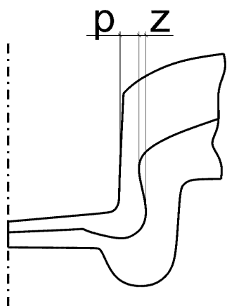
Rys. 2. Parametry geometryczne połączenia przetłaczanego [3]
