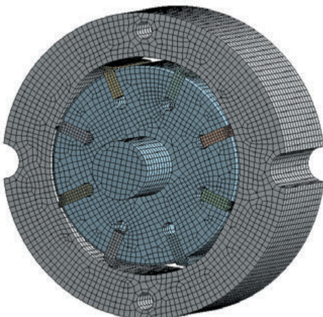
Rys. 4. Model MES pompy łopatkowej
