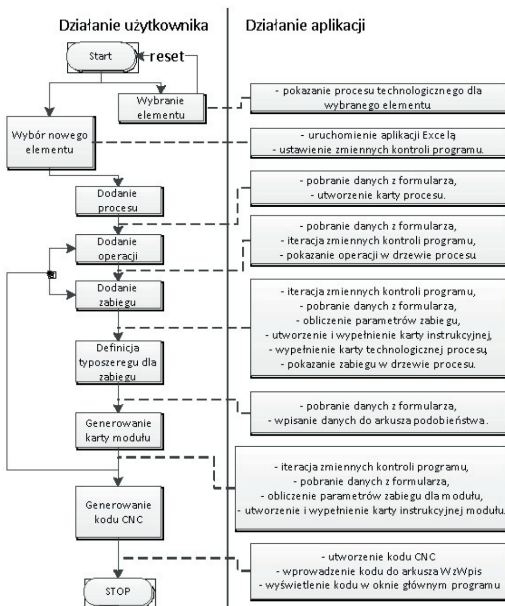
Rys. 4. Ogólny algorytm działania programu
