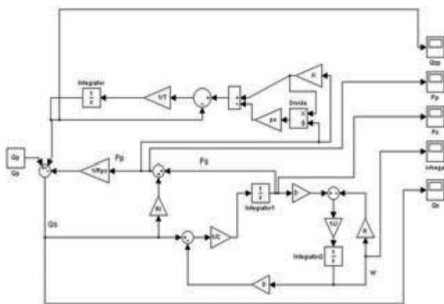
Rys. 5. Schemat blokowy układu
