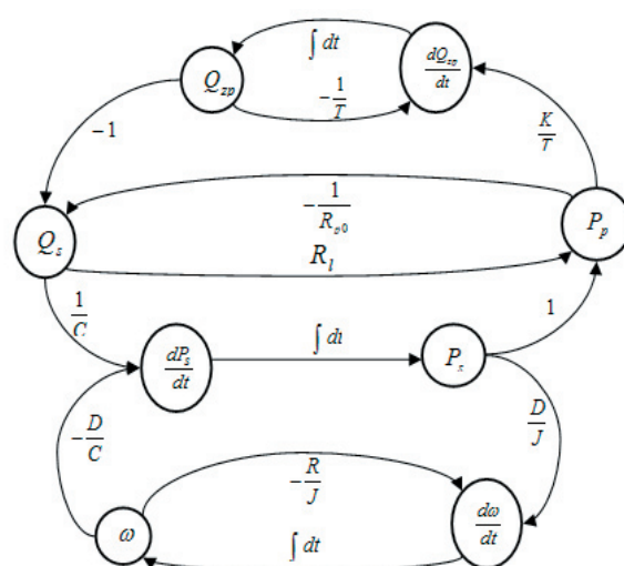
Rys. 6. Graf zależności przepływu sygnałów
