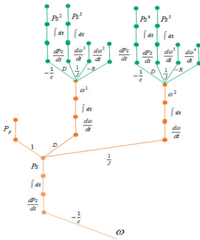
Rys. 14. Złożoność decyzyjna fragmentu 4 kompleksowej struktury S_{G\omega} z rysunku 12
