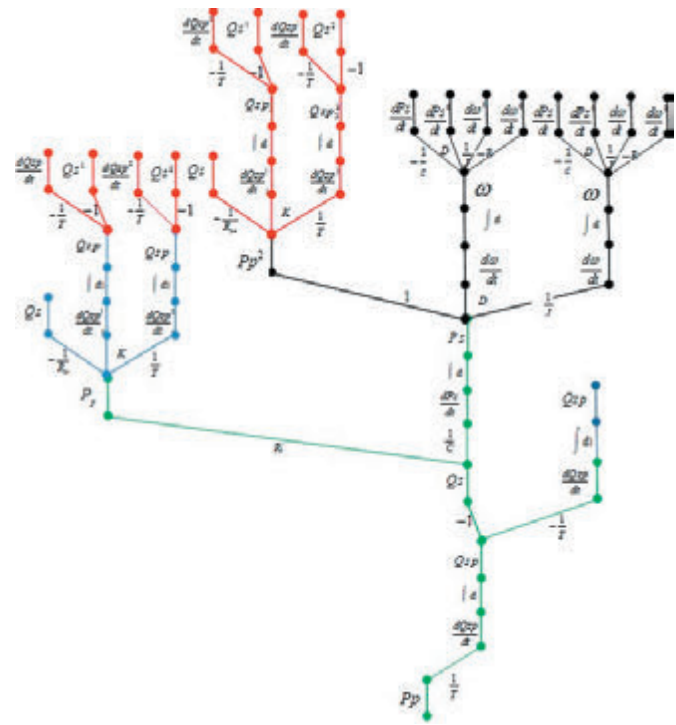
Rys. 15. Złożoność decyzyjna fragmentu 3 kompleksowej struktury S_{G\omega} z rysunku 12
