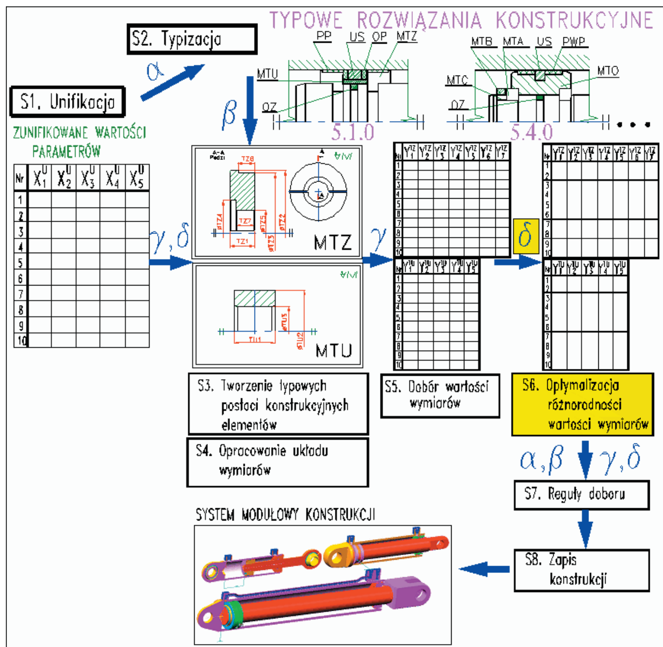
Rys. 1. Model przyporządkowań między cechami w uporządkowanych rodzinach konstrukcji
