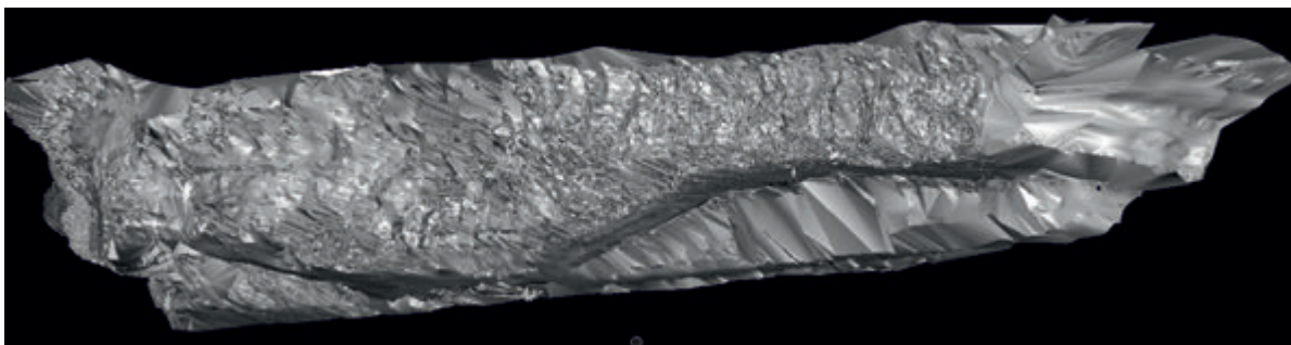
Rys. 6. Odwzorowanie numeryczne ściany eksploatacyjnej Fig. 6. Numerical model of wall
