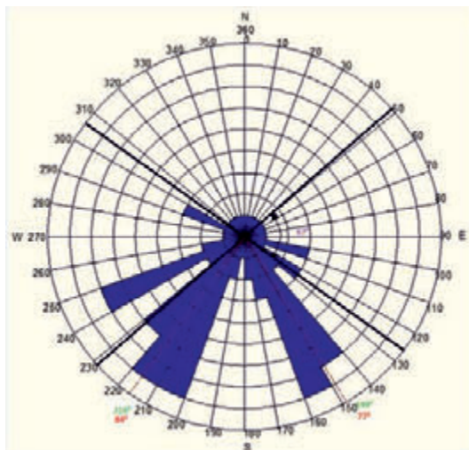
Rys. 1. Róża spękań ściany wyrobiska
