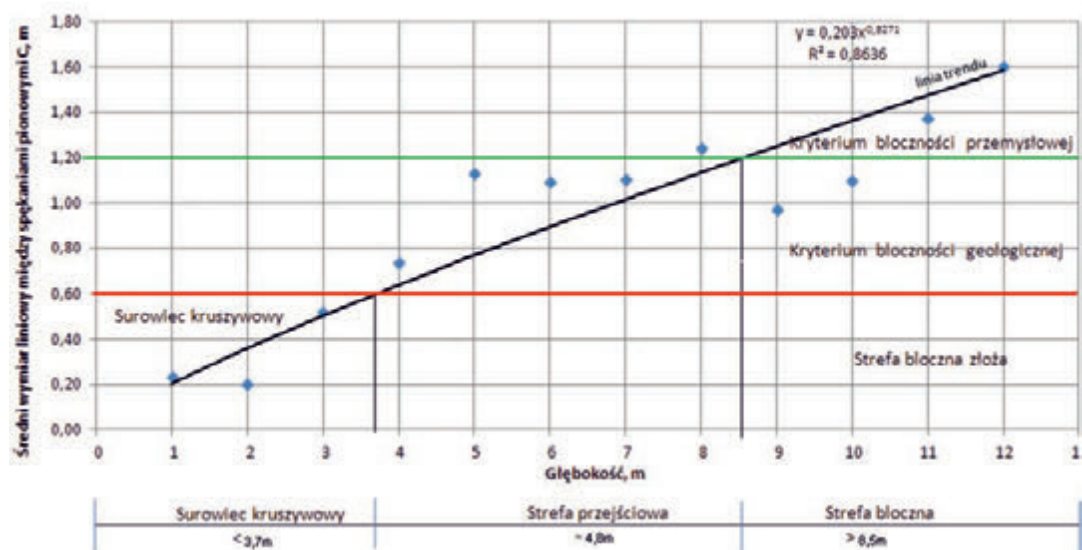
Rys. 9. Wyniki zmian naturalnej bloczności w funkcji głębokości zalegania
