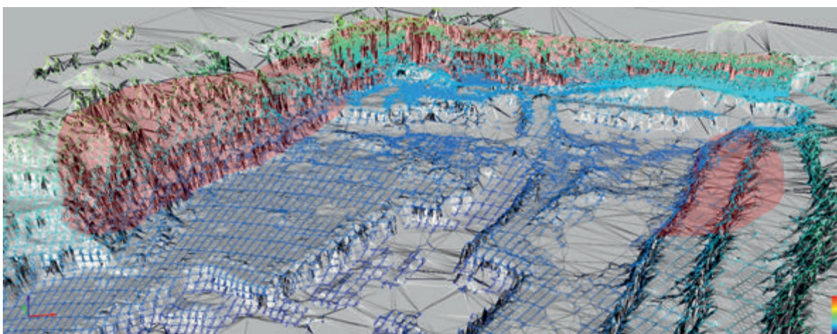
Rys. 5. Wizualizacja wyrobiska z wyodrębnionymi partiami blocznymi Fig. 5. Visualization of mining excavation with parties of block separateness
