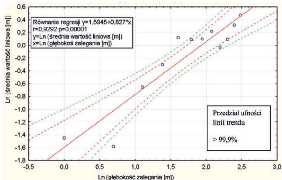
Rys. 8. Analiza trendu zmienności bloczności złoże
