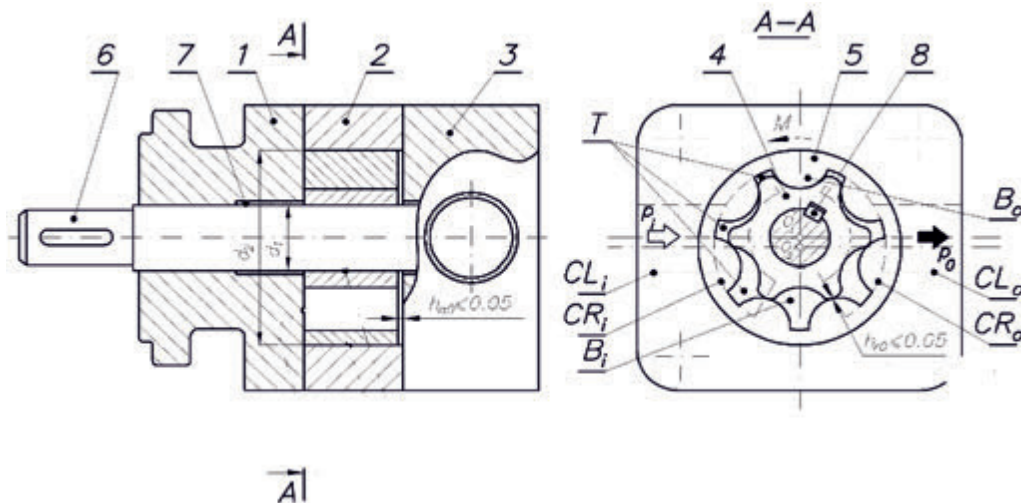
Rys. 2. Eksperymentalna pompa gerotorowa; 1,2,3 – części korpusu, 4,5 – koła zębate, 6 – wał napędowy, 7-łożysko, 8 – wpust T – komory międzyzębne, CL_i , CR_i , B_i – kanał, komora i mostek wejściowy, CL_o , CR_o , B_o – kanał, komora i mostek wyjściowy, p_i – ciśnienie wejściowe, p_o – ciśnienie na wyjściu z pompy
