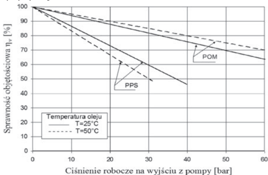
Rys. 10. Porównanie sprawności objętościowej pompy gerotorowej z kołami z POM i PPS
