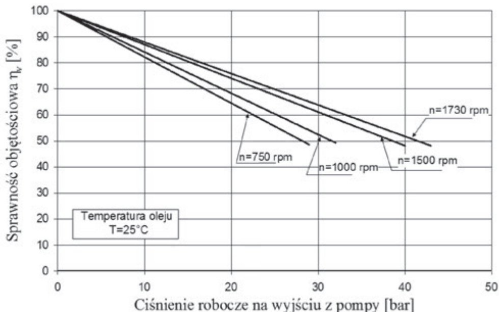
Rys. 9. Sprawność objętościowa pompy z kołami wykonanymi z PPS
