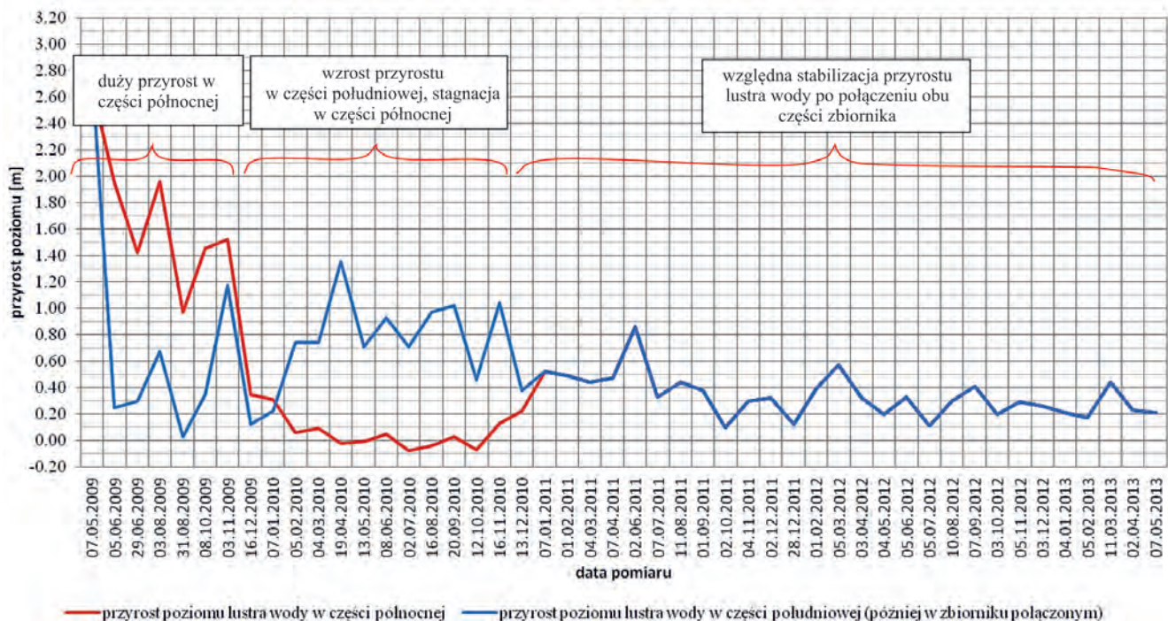
Rys. 4. Obserwowany przyrost zwierciadła wody w zbiorniku Lubstów
