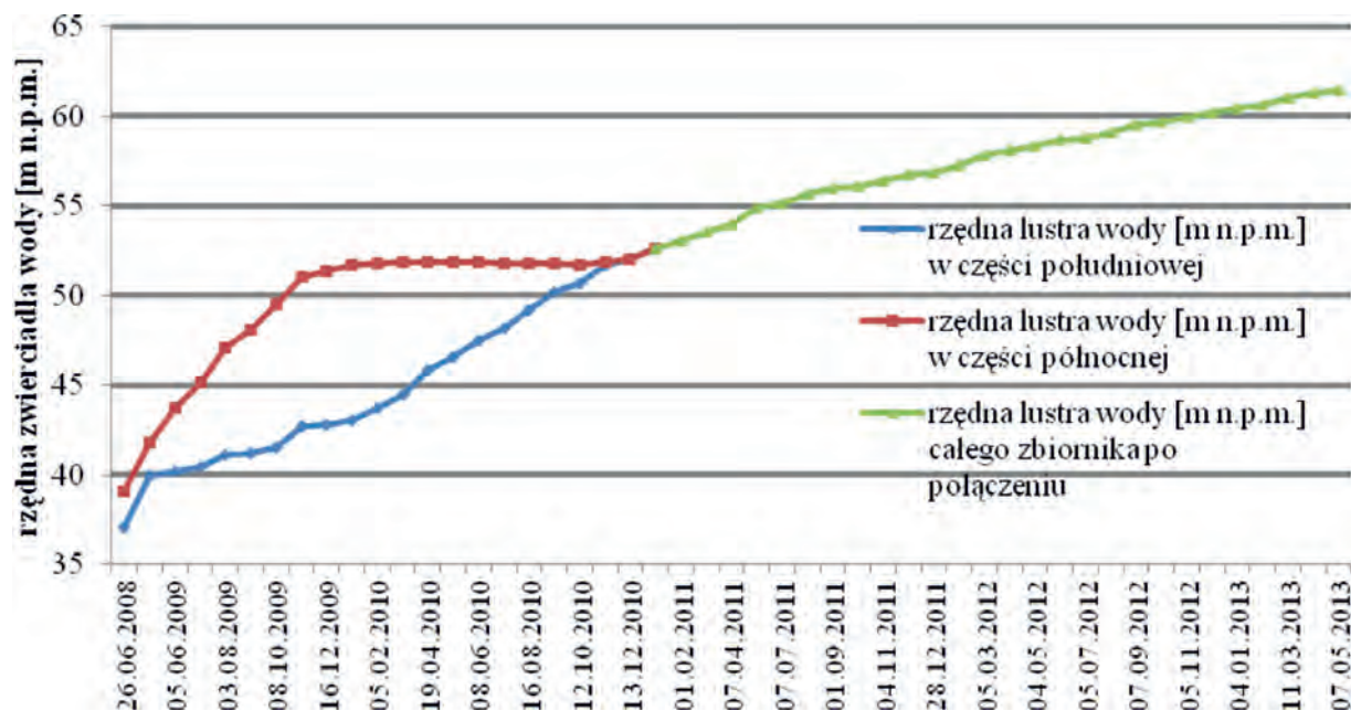
Rys. 3. Pomiar rzeczywistych rzędnych zwierciadła wody w budowanym zbiorniku Lubstów w okresie 2008 – 2013
