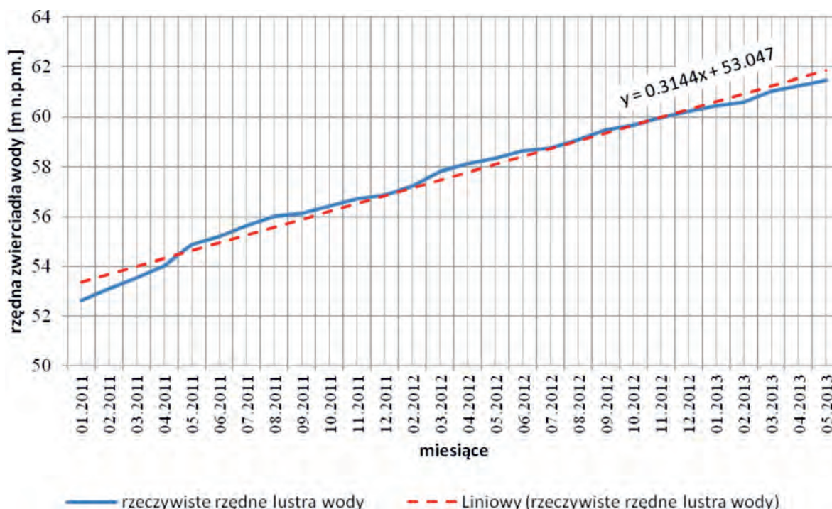
Rys. 5. Rzeczywiste rzędne zwierciadła wody wraz z linią trendu
