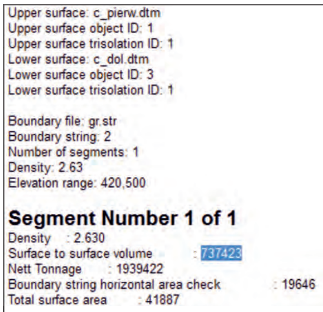
Rys. 11. Fragment raportu obliczenia objętości pomiędzy płaszczyznami: spągu i pierwotną
