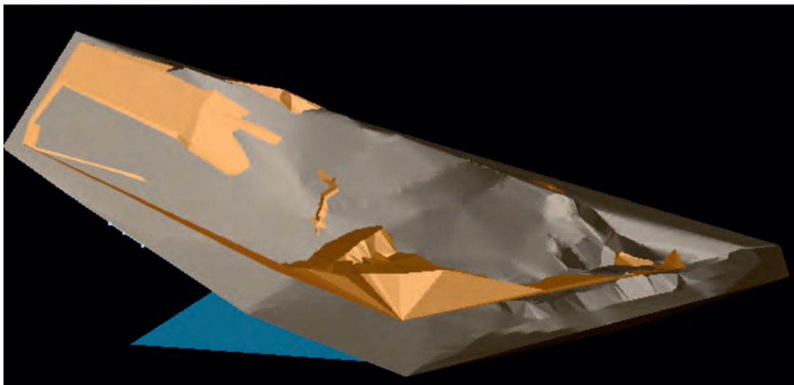
Rys. 9. Numeryczne modele terenu: spąg pokładu, stan pierwotny i stan na dzień pomiarów Fig. 9. DTM of the strata floor: primary geometry and actual
