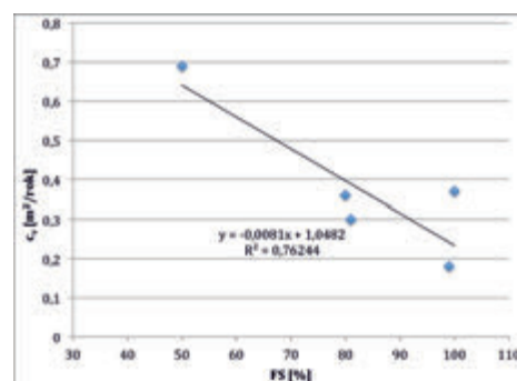
Rys. 4. Zależność pomiędzy współczynnikiem konsolidacji c_v a pęcznieniem swobodnym FS
