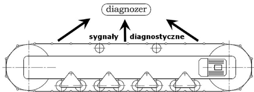
Rys. 2. Schemat diagnozowania podwozi gąsienicowych zewnętrznym testerem
