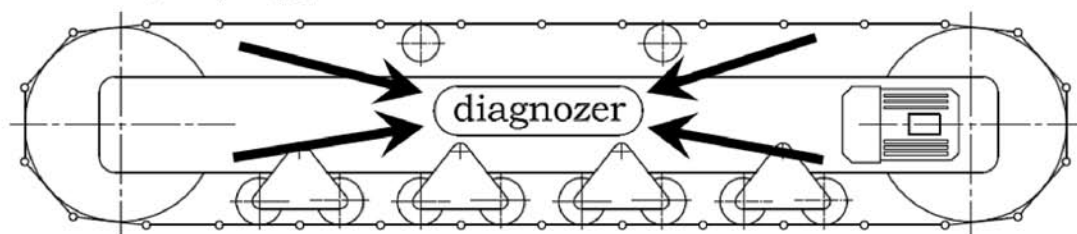
Rys. 3. Schemat diagnozowania podwozi gąsienicowych wewnętrznym testerem umieszczonym na elemencie nieruchomym Fig. 3. Diagram of caterpillar chassis diagnosis with internal tester located at immobile element
