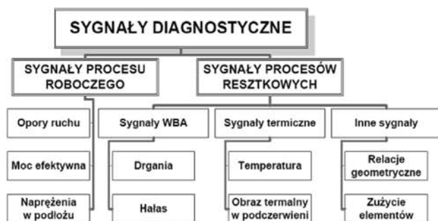
Rys. 1. Sygnały diagnostyczne do oceny stanu technicznego podwozi gąsienicowych (opracowanie własne na podstawie [16, 17])
