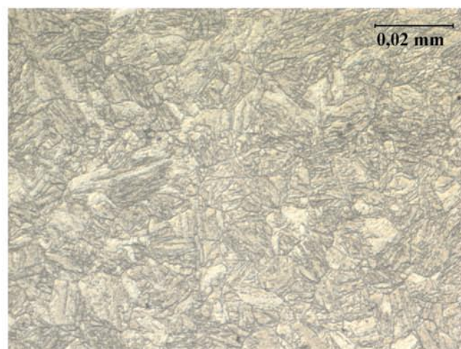
Rys.12. Próbką 4. Iglasta mikrostruktura odpuszczania o orientacji pomartenzycyjnej. Pow.1000x, trawiono MilFe, mikroskopia świetlna
