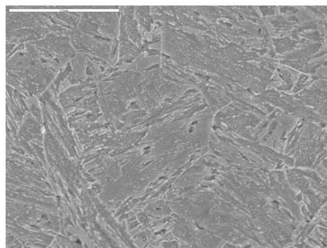
Rys.13. Próbką 4. Struktura odpuszczonego martenzytu z pojedynczymi, drobnymi, częściowo skoagulowanymi wydzieleniami węglkowymi. Pow.4500x, trawiono MilFe, SEM
