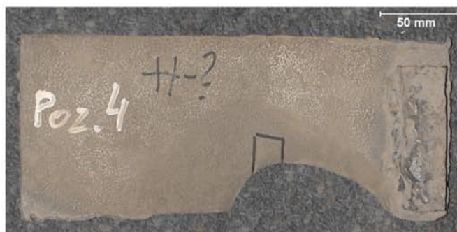
Rys.4. Próbka 4. Makroskopowy obraz blachy wykładzinowej osłaniającej konstrukcję przesypu. Grubość początkowa 15 mm, uziarnienie materiału melaufirowego 16 – 22 mm, czas pracy około 1350 godzin, przerób około 35 000 ton
