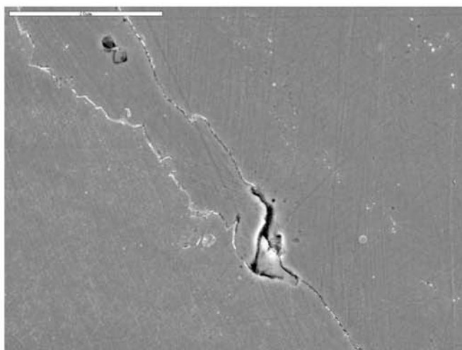
Rys.10. Próbką 2. Granice ziaren austenitu z ciągłą otoczką węglkową. U zbiegu granic widoczna mikronieciągłość struktury na granicy międzyfazowej węglk (Fe,Mn)3C – austenit. Pow.2200x, trawiono MilFe, SEM
