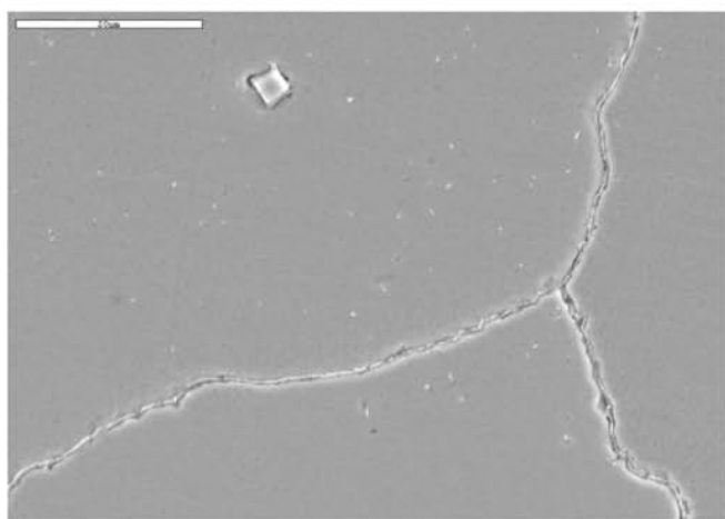
Rys.8. Próbką 1. Zbieg granic ziaren austenitu udekorowany ciągłą otoczką wydzielen węglkowych. Widoczny także duży, pojedynczy węglk w obszarze ziarna. Pow.1000x, trawiono MilFe, SEM
