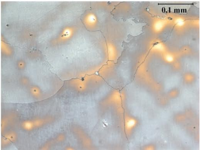
Rys.7. Próbka 2. Mikrostruktura austenitu stopowego z wydzieleniami cementytu manganowego głównie na granicach i u zbiegu ziaren. Pow.200x, trawiono MilFe, mikroskopia świetlna Fig. 7. Sample 2. Alloying austenite microtexture with manganese cementite precipitations mainly at grains boundaries and junctions. Magnification of 1x 200, etched with MilFe, light microscopy (LM)
