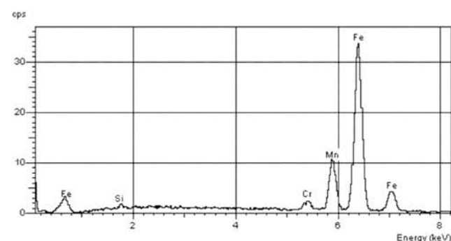
Rys.9. Próbką 1. Widmo energetyczne promieniowania rentgenowskiego z obszaru próbki pokazanej na rys.8
