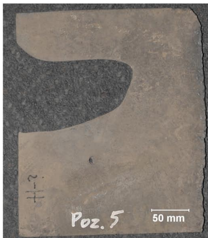
Rys.5. Próbką 5. Makroskopowy obraz blachy wykładzinowej przesyłu drobnego kruszcu melaforowego (uziarnienie 4 – 35 mm, ostrokrawędziowy, czas pracy około 1400 godzin, przerób około 70 000 ton)
