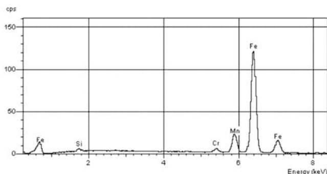
Rys.11. Próbką 2. Widmo energetyczne promieniowania rentgenowskiego z obszaru próbki pokazanej na rys.10
