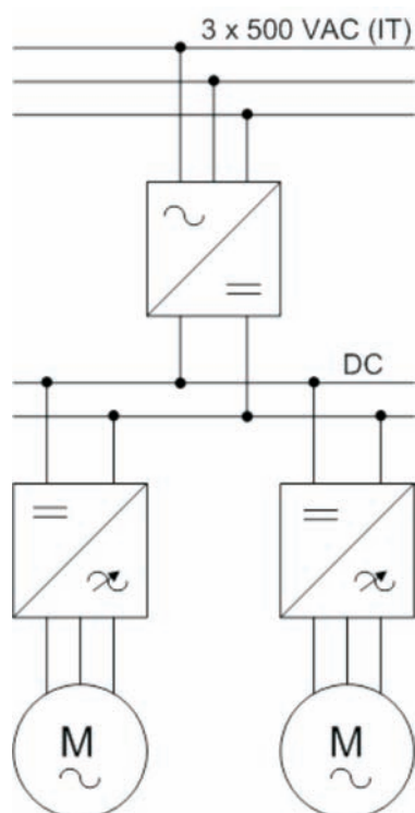
Rys. 1. Ogólny schemat układu zasilania i sterowania przenośników taśmowych Z-3B i Z-4B
