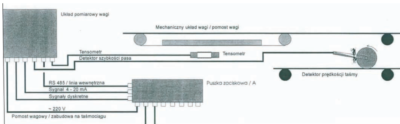
Rys. 2. Schemat ideowy układu wagi zainstalowanej na przenośniku Z2B do regulacji prędkości obrotowej przenośników Z-3B i Z4B
