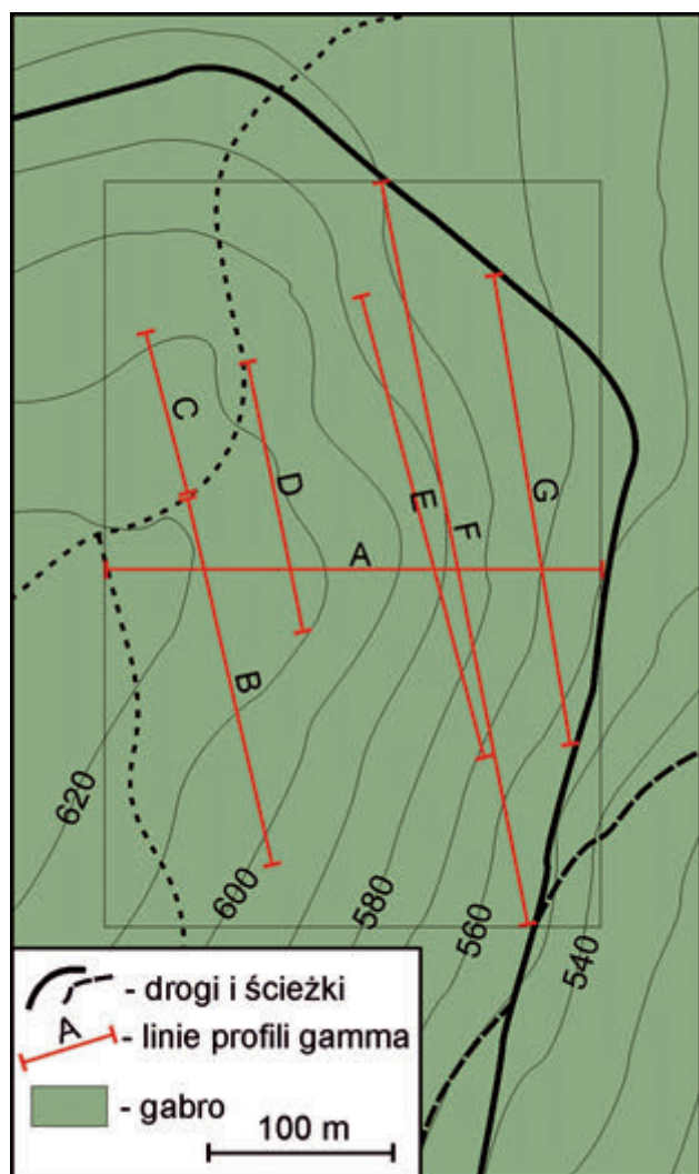
Rys. 5. Przebieg linii profilowania gamma na poligonie doświadczalnym Fig. 5. Gamma profiles on the test polygon (with ilmenite body)
