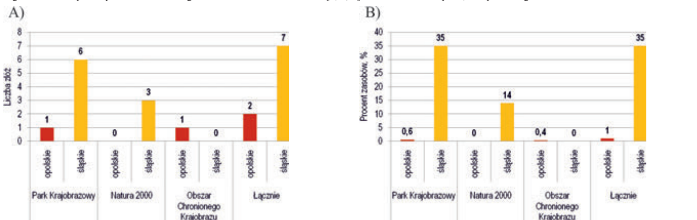
Rys. 6. Niezagospodarowane złoża kamieni łamanych i blocznych w obszarach przyrodniczo cennych A – liczba złóż, B – procent zasobów bilansowych [3, 4, 5]
