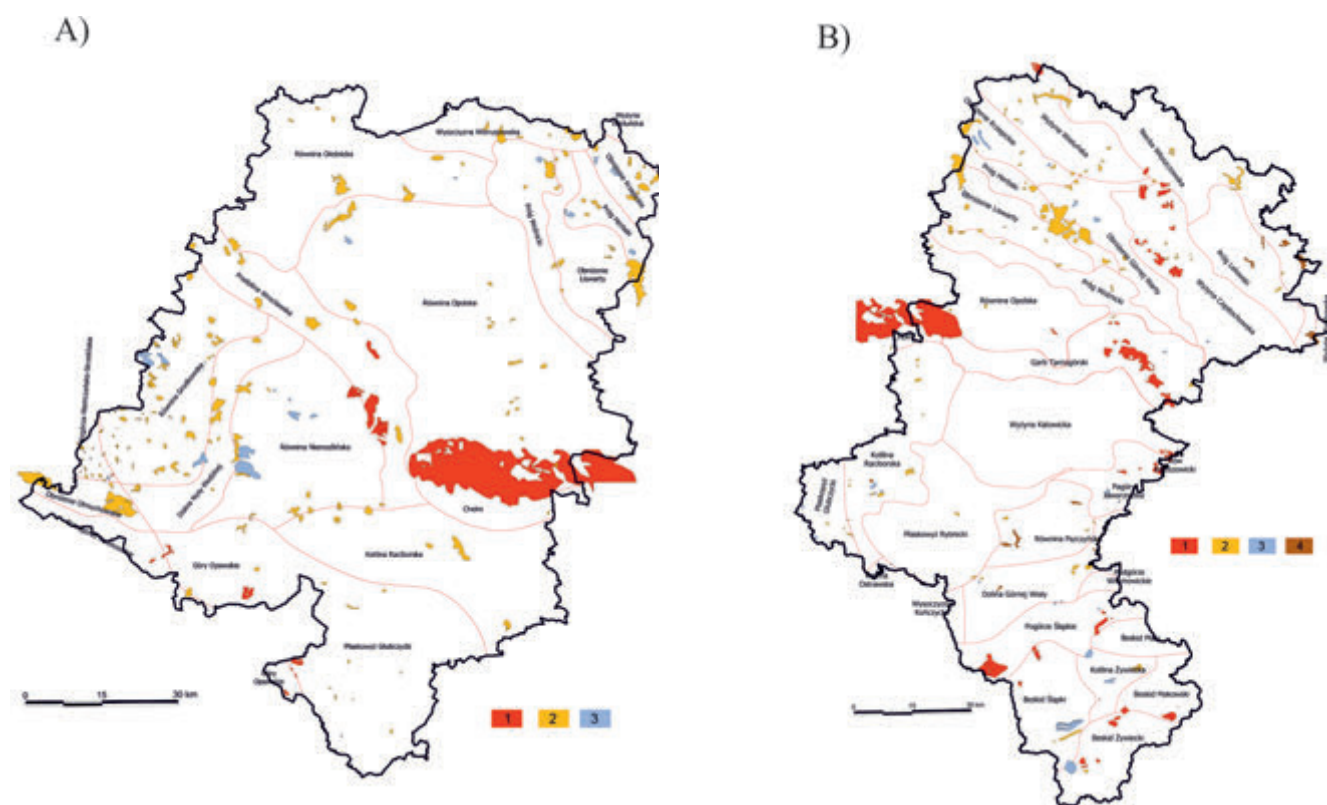
Rys. 3. Rozmieszczenie obszarów perspektywicznych dla udokumentowania złóż surowców mineralnych w województwie opolskim (A) i śląskim (B) [2]
