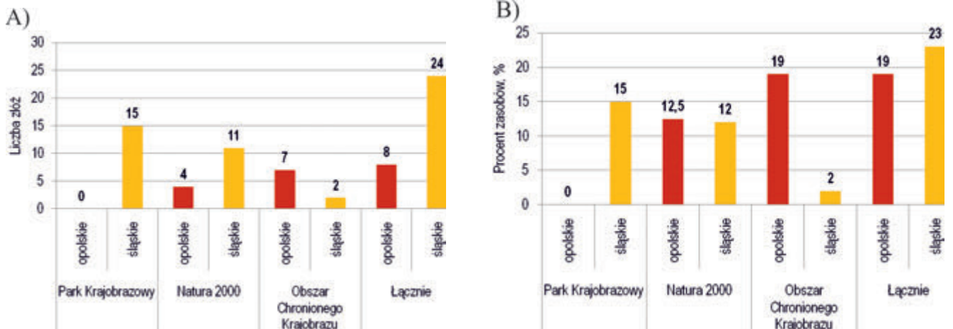
Rys. 5. Niezagospodarowane złoża piasków i żwirów w obszarach przyrodniczo cennych [3, 4, 5] A – liczba złóż, B – procent zasobów bilansowych Fig. 5. Undeveloped deposits of sand and gravel in valuable natural areas [3, 4, 5] A – number of deposits, B – percentage of resources
