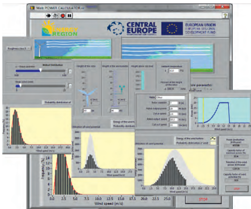
Rys. 1. Panel czołowy programu PowerCalculator (zakładki: warunki wietrzności, wysokość turbiny, turbina)
