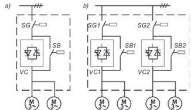
Rys. 2. Tyrystorowe układy łagodnego rozruchu napędów wielosilnikowych: a) do jednoczesnego rozruchu 2 silników; b) zintegrowany układ z dwoma sterownikami we wspólnej obudowie (VC - tyrystorowy sterownik napięcia; SG - stycznik główny, SB - stycznik by-pass)
