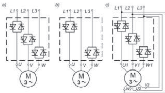
Rys. 1. Przekształtnikowe układy płynnego rozruchu o sterowaniu fazowym: a), b) - układy In Line ; c) - układ In Delta
