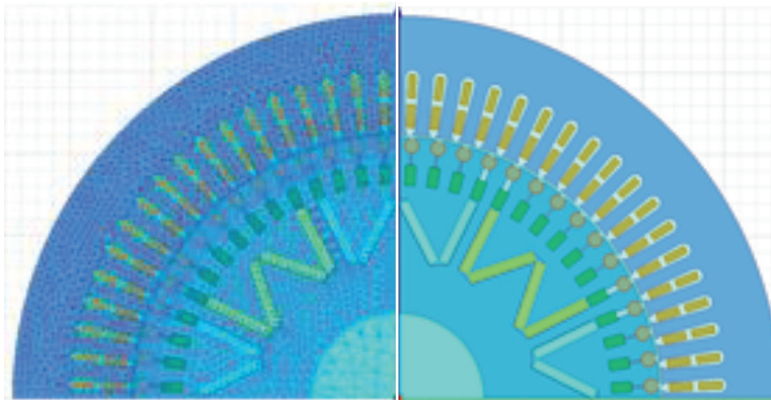
Rys. 1. Geometria części połowej rozpatrywanego modelu silnika Fig. 1. Field part geometry of studied LSPMSM
