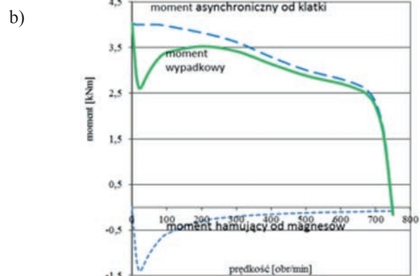
Rys. 2. Charakterystyka prądu rozruchowego stojana (a) oraz momentu silnika (b) w funkcji prędkości obrotowej Fig. 2. Characteristics of current vs. speed (a) and torque vs. speed (b)
