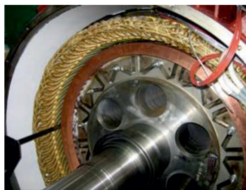
Rys. 4. Widok wirnika z magnesami trwałymi o mocy P=1100 kW Fig. 4. A picture of the fabricated rotor of 1100 kW LSPMSM
