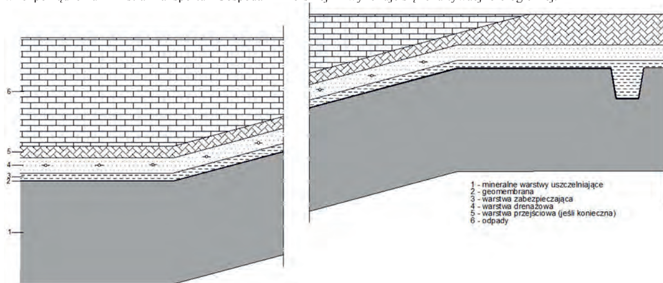
Rys. 1. Profil składowiska odpadów i sposób zakotwienia geomembrany (oprac. własne na podstawie [2, 7])
