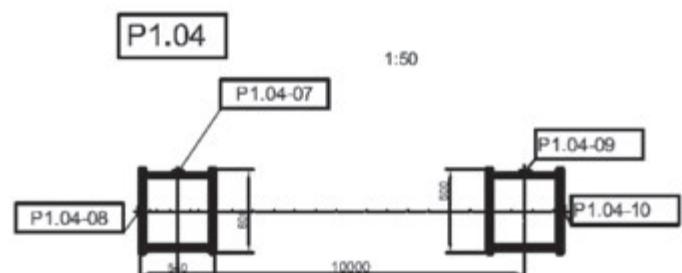
Rys. 6. Punkty pomiarowe na dźwigarze wysięgnika koła czerpakowego w okolicy przegubu zwodzenia
