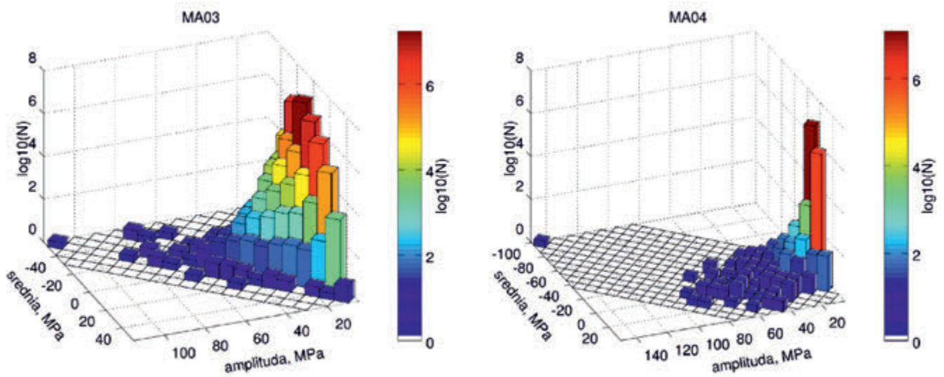
Rys. 3b. Rozkład amplitud maksymalnych (MPa), ich wartość uśredniona (MPa) oraz ich licznosc występowania (logN) w czasie trwania badań – punkty MA03 i MA04
