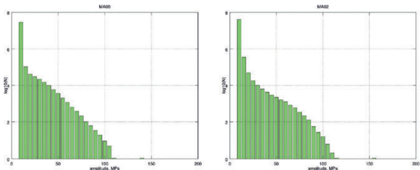
Rys. 2a. Rozkład amplitud maksymalnych (MPa) oraz ich licznosc występowania ( \log N ) w czasie trwania badań – punkty MA00 i MA02
