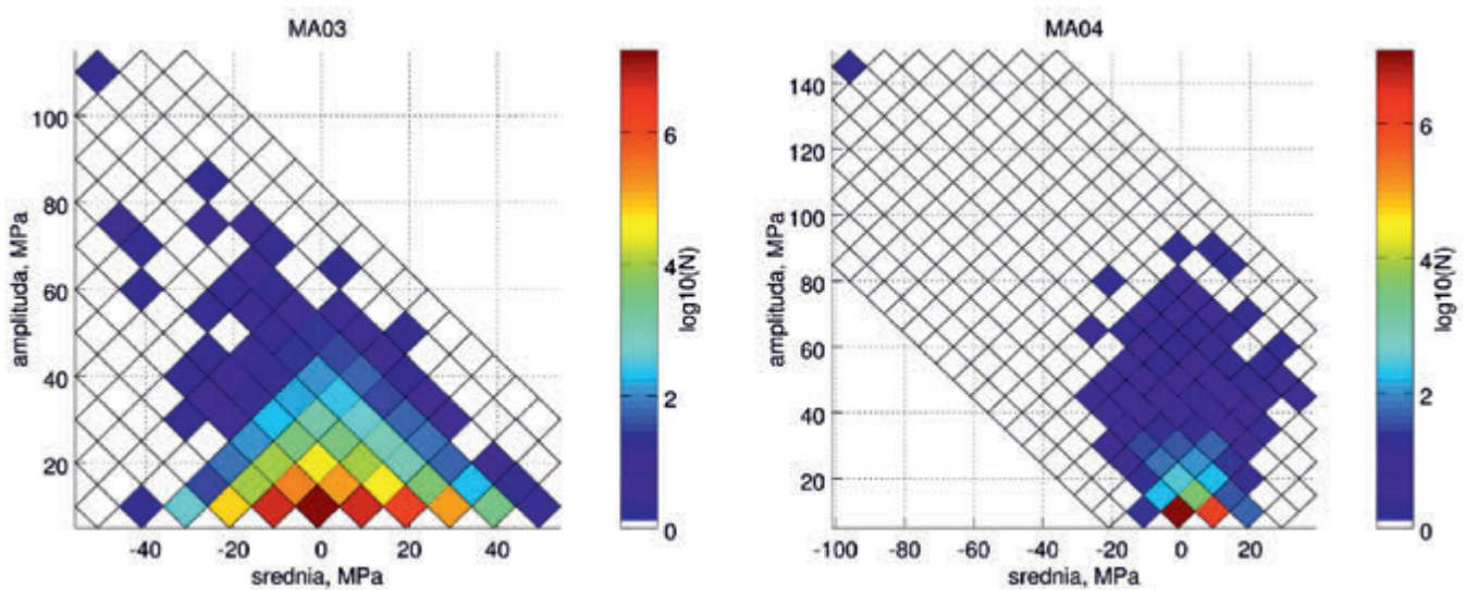
Rys. 3c. Rozkład amplitud maksymalnych w funkcji wartości średnich – punkty MA03 i MA04
