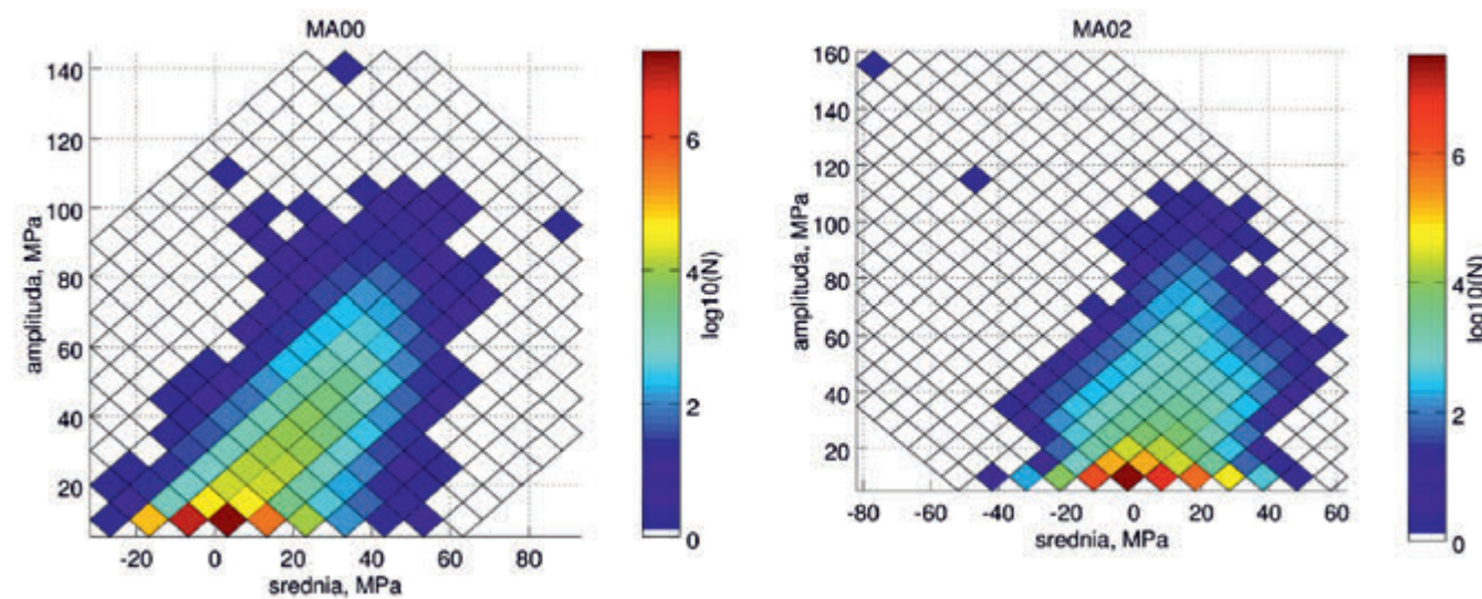
Rys. 2c. Rozkład amplitud maksymalnych w funkcji wartości średnich – punkty MA00 i MA02
