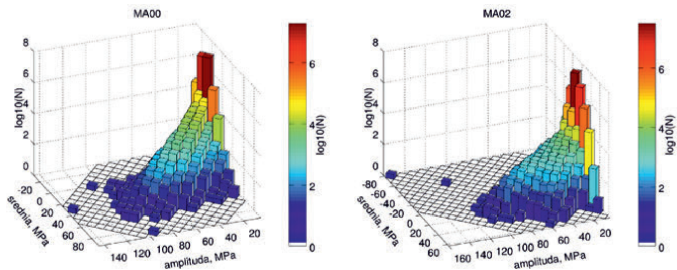
Rys. 2b. Rozkład amplitud maksymalnych (MPa), ich wartość uśredniona (MPa) oraz ich licznosc występowania ( \log N ) w czasie trwania badań – punkty MA00 i MA02
