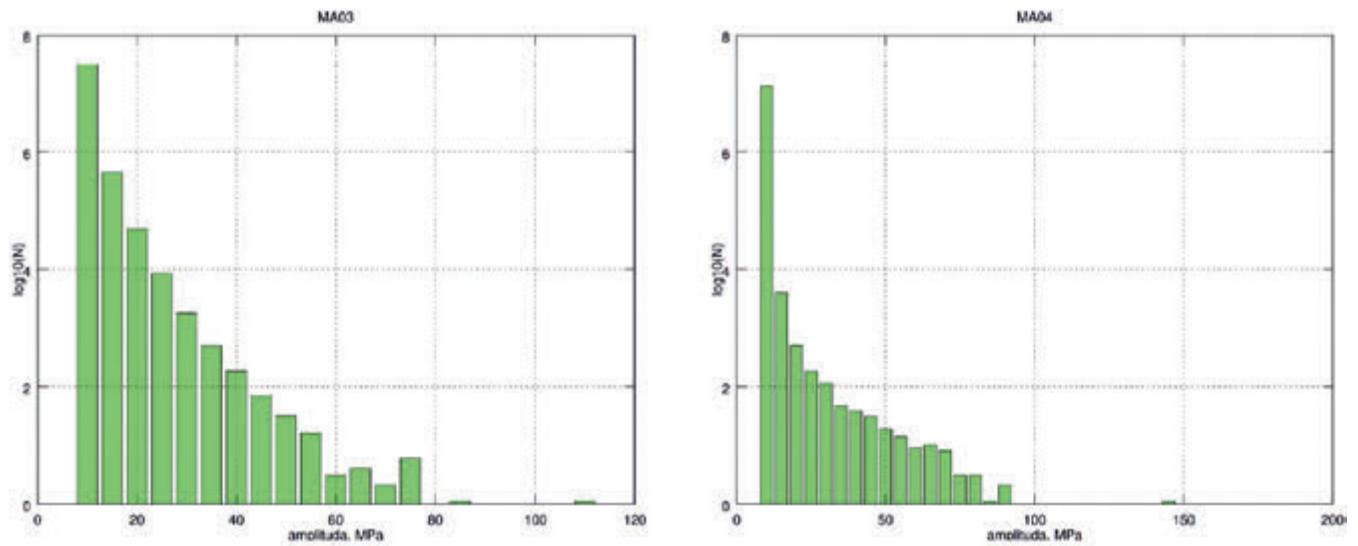
Rys. 3a. Rozkład amplitud maksymalnych (MPa) oraz ich licznosc występowania (logN) w czasie trwania badań – punkty MA03 i MA04
