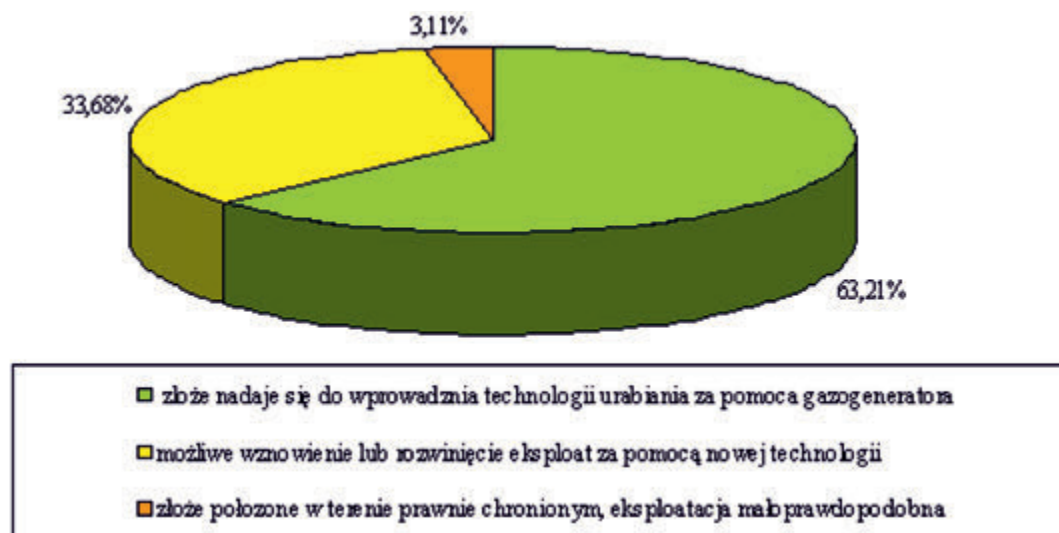
Rys. 4. Podział polskich złóż blocznych pod względem możliwości zastosowania gazogeneratora
