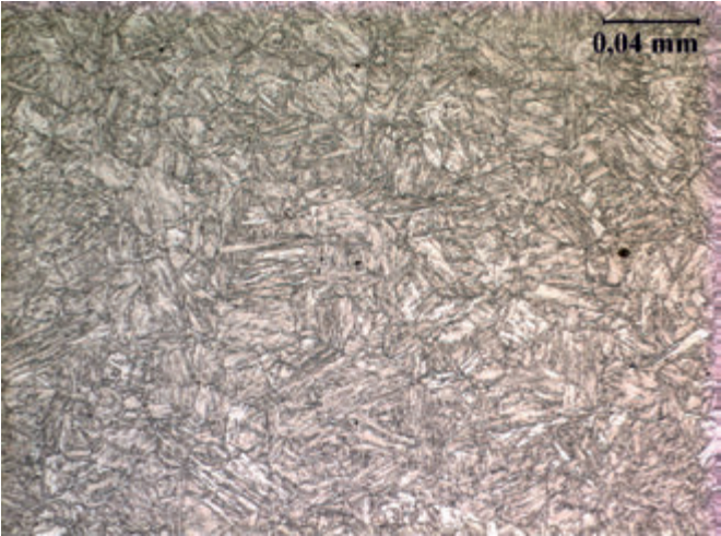
Rys. 5. Mikrostruktura blachy o grubości 12 mm ze stali Weldox 700Struktura niskowęglowego martenzytu. Trawiono Mi1Fe Fig. 5. Microstructure of the sheet gauge 12 mm made from Weldox 700 steel. Structure of the low-carbon martensite. Etched with Mi1Fe
