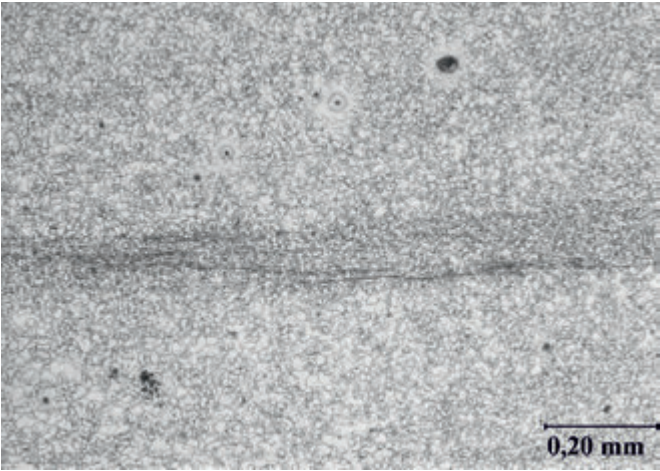
Rys. 4. Mikrostruktura stali Weldox 700 o grubości blachy 8 mm. Drobnziarnista struktura ferrytyczna z widoczną segregacją węglików w środkowej części blachy. Trawiono Mi1Fe Fig. 4. Microstructure of the sheet gauge 8 mm made from Weldox 700 steel . Ferritic structure with segregation of carbides in middle part of the sheet. Etched with Mi1Fe
