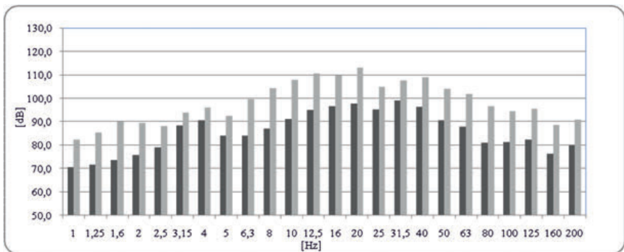
Rys. 5. Wyniki pomiarów hałasu niskoczęstotliwościowego w kabinie wiertnicy samojedznej
