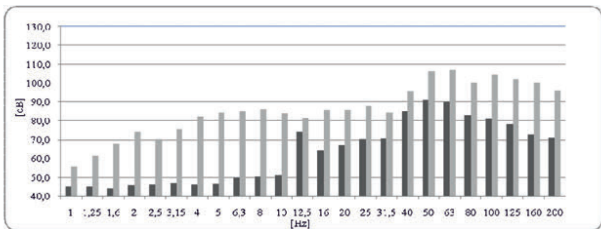
Rys. 6. Wyniki pomiarów hałasu niskoczęstotliwościowego w kabinie dźwigu samojedznego
