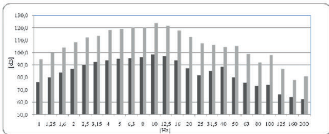
Rys. 1. Wyniki pomiarów hałasu niskoczęstotliwościowego w kabinie ładowarki
