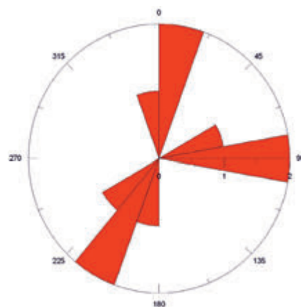
Pokłady 416/1 i 416/1-2 Seams 416/1 and 416/1-2
