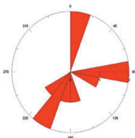
Pokłady 418/1 i 418/1-2 Seams 418/1 and 418/1-2
