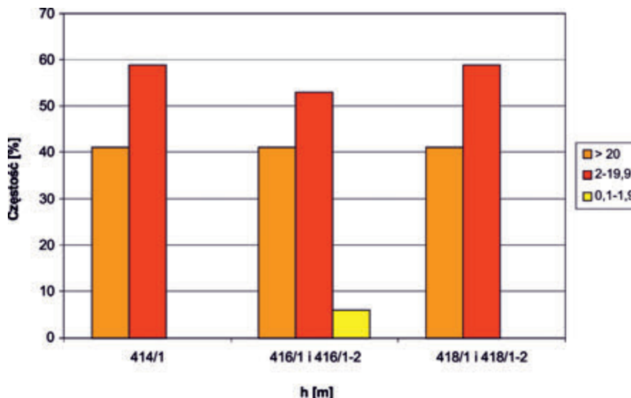
Rys. 4. Rozkład wielkości zrzutu wszystkich uskoków (h) w wydzielonym obszarze zagospodarowanym dla pokładów 414/1, 416/1 i 416/1-2, 418/1 i 418/1-2 Fig. 4. Distribution of the throw of faults (h) in a set area of the exploited field seams 414/1, 416/1 and 416/1-2, 418/1 and 418/1-2
