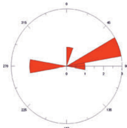
Pokład 414/1 Seam 414/1
