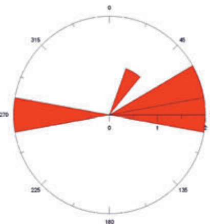
Pokłady 418/1 i 418/1-2 Seams 418/1 and 418/1-2
