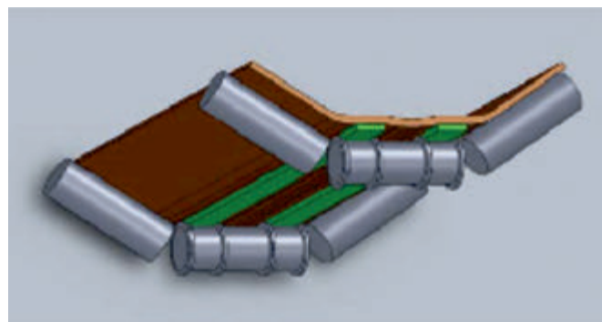
Rys. 3.a) Lina pędna typu SAG 2,5- 65 x 22/2x9 -1770, b) koncepcja prowadzenie lin pędnych z zastosowaniem pierścieni ustalających na krążniku [Gładysiewicz 2013]
