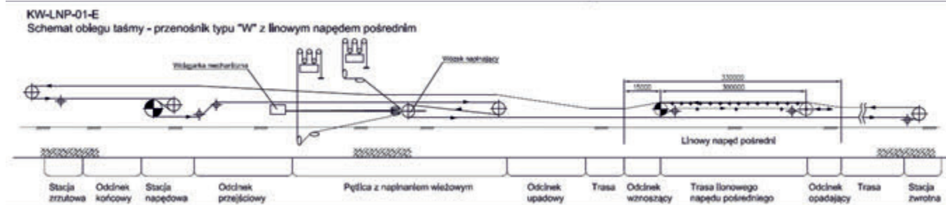
Rys. 5. Schemat obrotu taśmy na prototypowym przenośniku L_{NP} LEGMET (Gładysiewicz 2013)
